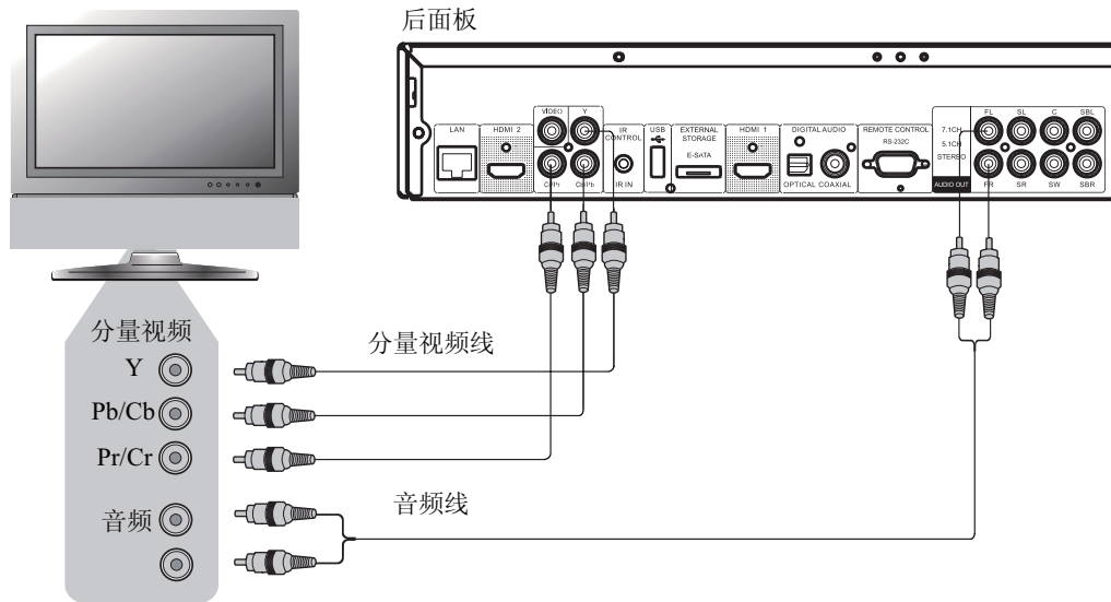
方法 4 –分量视频与电视机的连接
