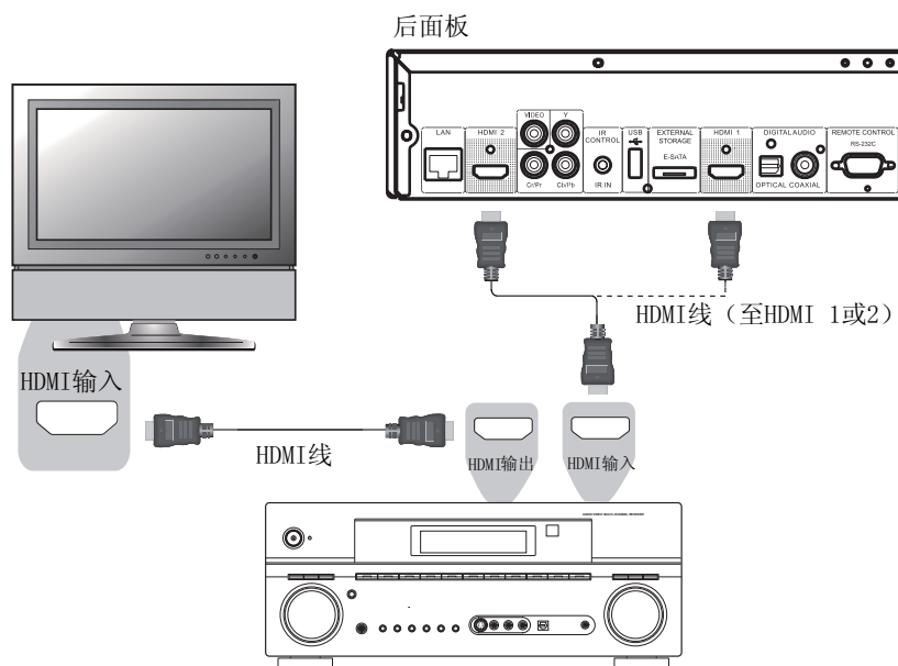
方法 5– HDMI 与功放和电视机的连接
