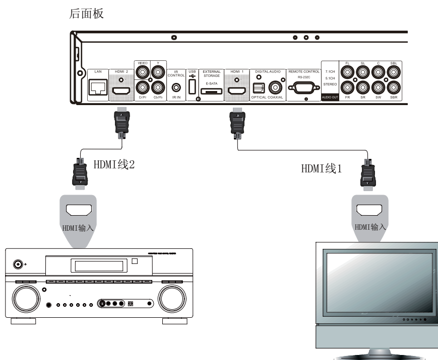
方法 9 – 双 HDMI 连接
