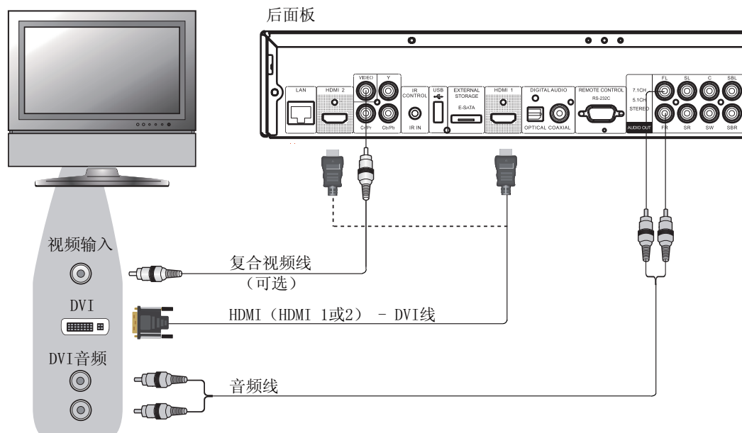
方法 3 – DVI 与电视机连接
