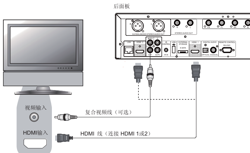
方法 1 – HDMI 直接与一台电视机连接
