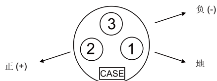
BDP-95 使用的公型平衡 XLR 端口
