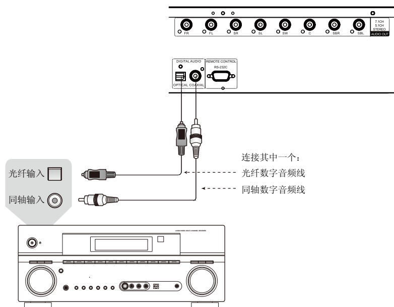
方法 7 – 数字音频连接
