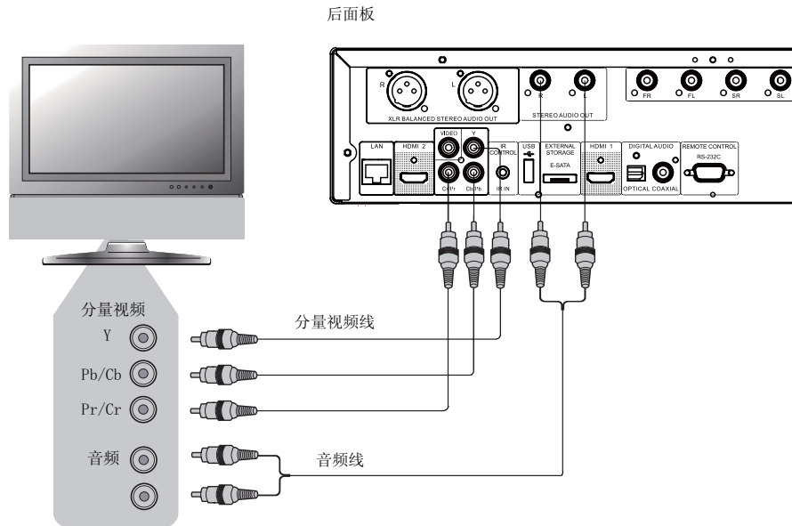
方法 4 –分量视频与电视机的连接
