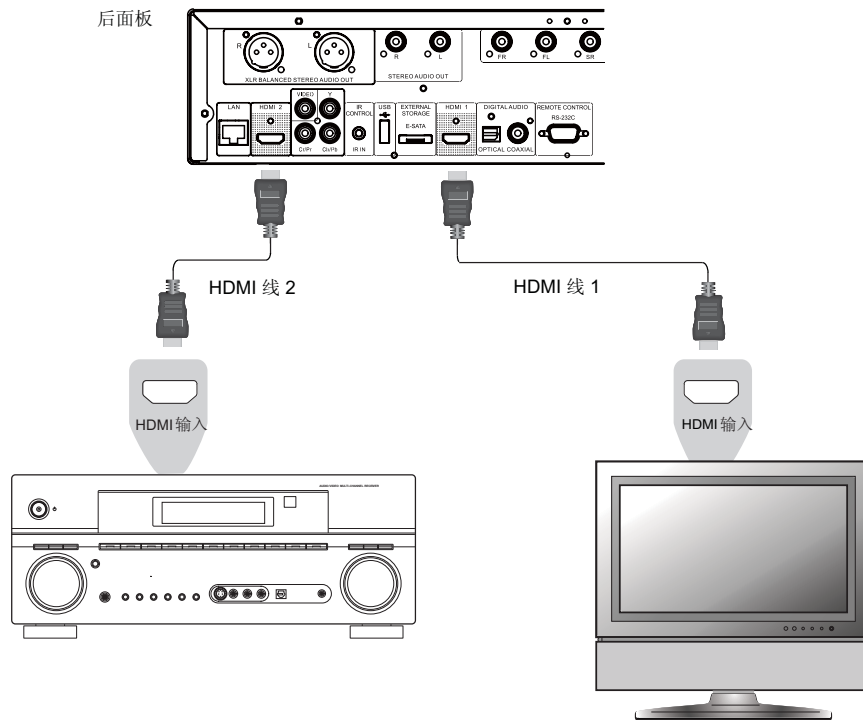
方法 10—双 HDMI 连接
