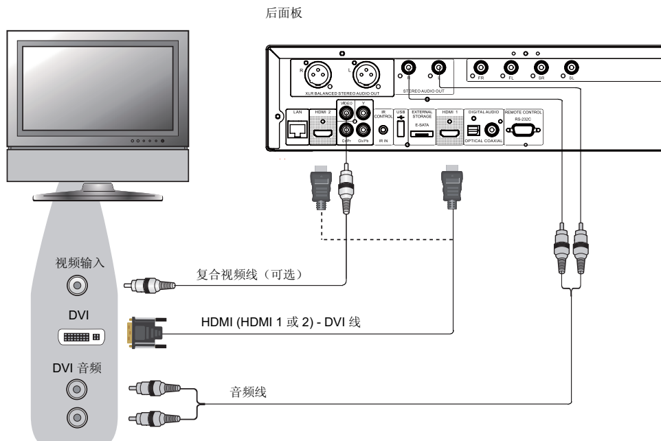
方法 3 – DVI 与电视机连接
