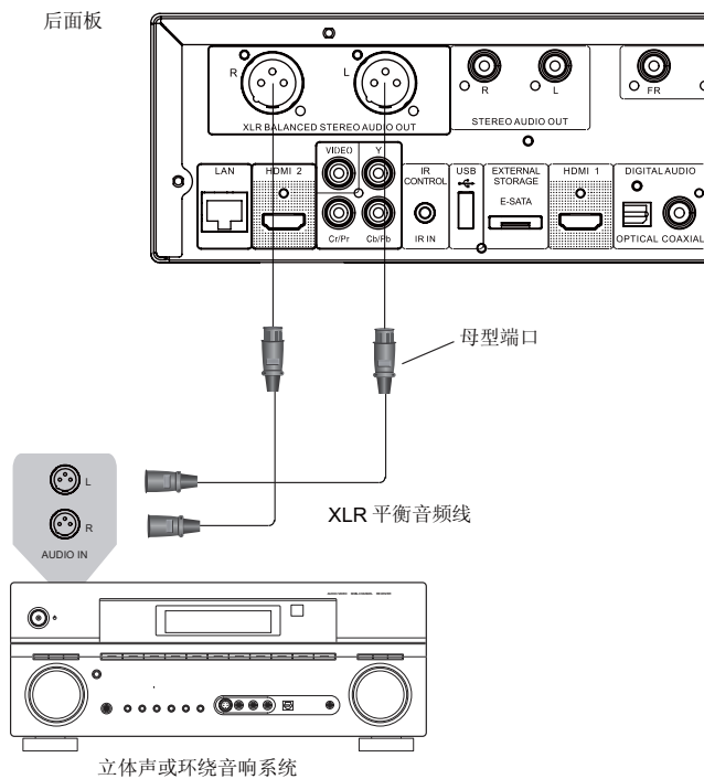
方法9 – 使用XLR平衡音频线连接到立体声音响系统
